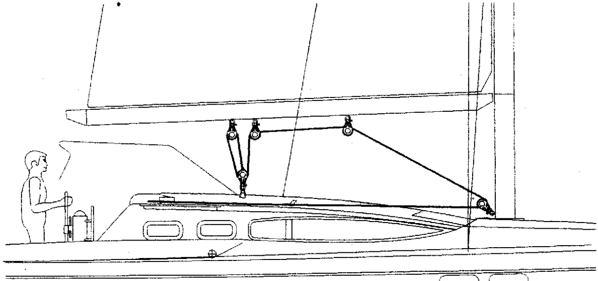
Retour de la drosse d'enrouleur de génois Genoa control line return
